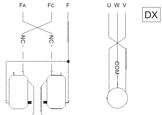
Блок микровыключателей Двигатель 220В
