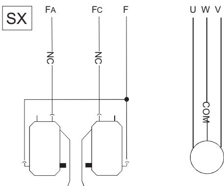
Блок микровыключателей Двигатель 220В
